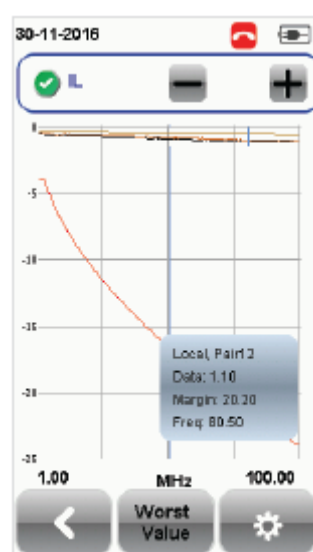
Вносимые потери
