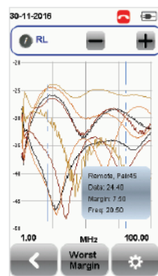
Обратные потери
