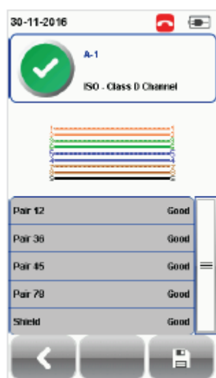
Разводка проводов
